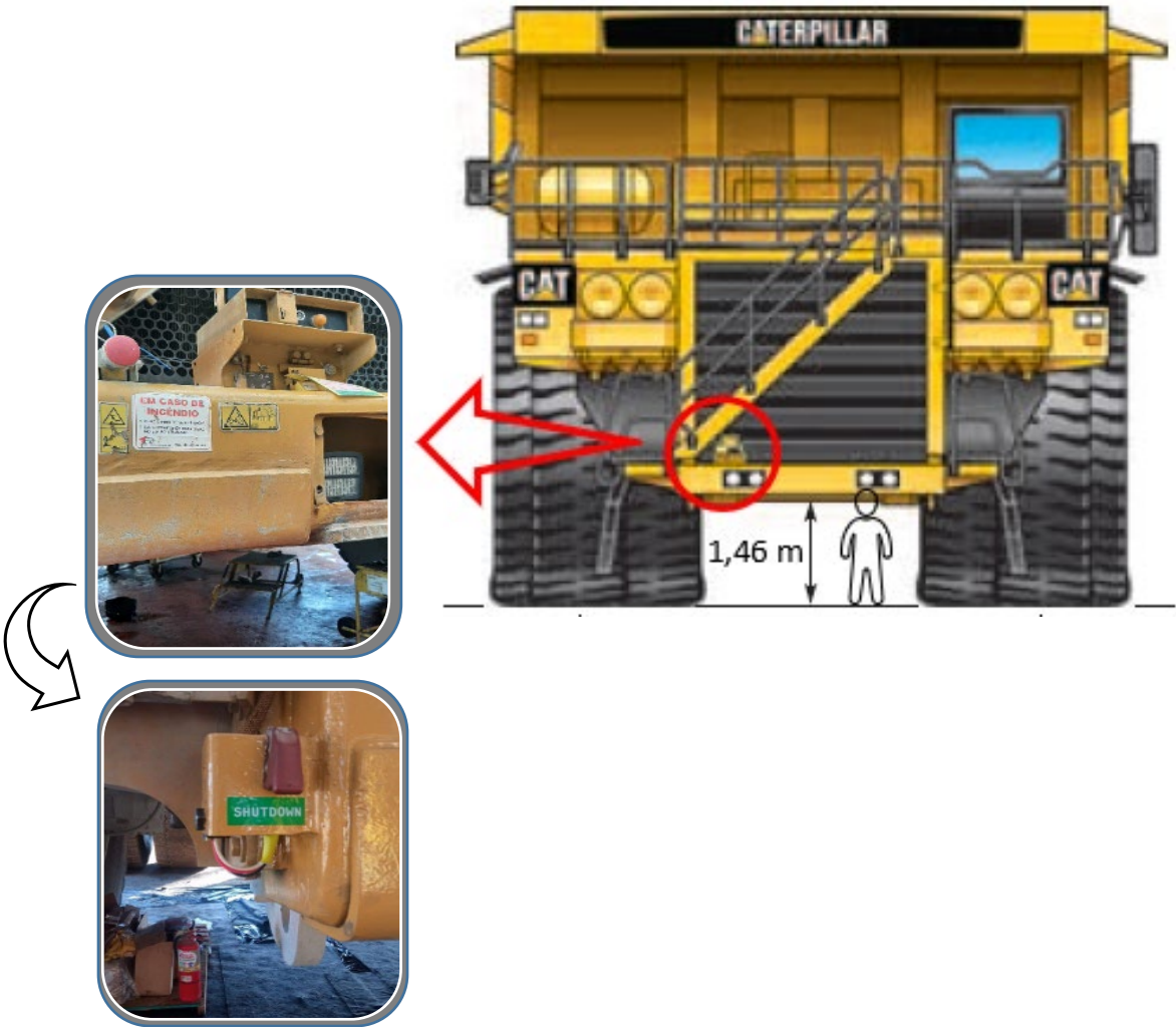
New shutdown switch position – Source: SOTREQ/Giesi Nascimento.
